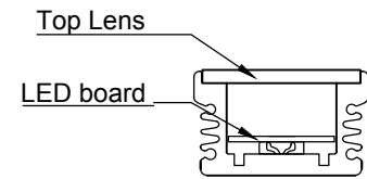
4 SECTION SCALE: 6"=1'-0"
