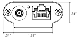
End Cap
