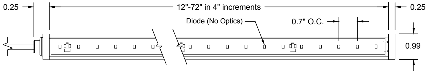
1 PLAN VIEW SCALE: 6"=1'-0"
