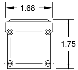
3 END CAP SCALE: 6"=1'-0"
