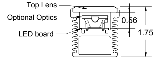
4 SECTION SCALE: 6"=1'-0"
