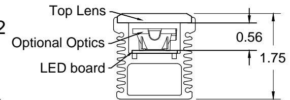
4 SECTION SCALE: 6"=1'-0"
